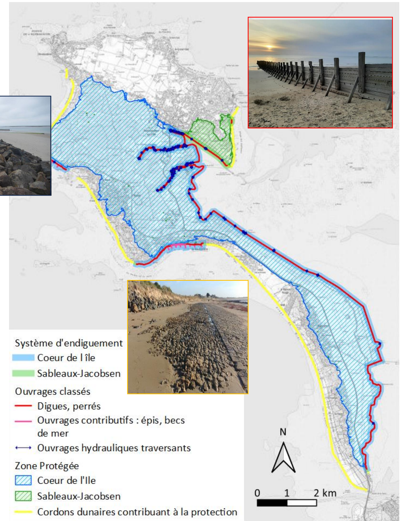
Systèmes d'endiguement de l'île de Noirmoutier
